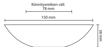
Mitat pohjakotelon kanssa (IP44)
