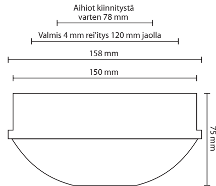
Mitat pohjakotelon kanssa (IP44)
